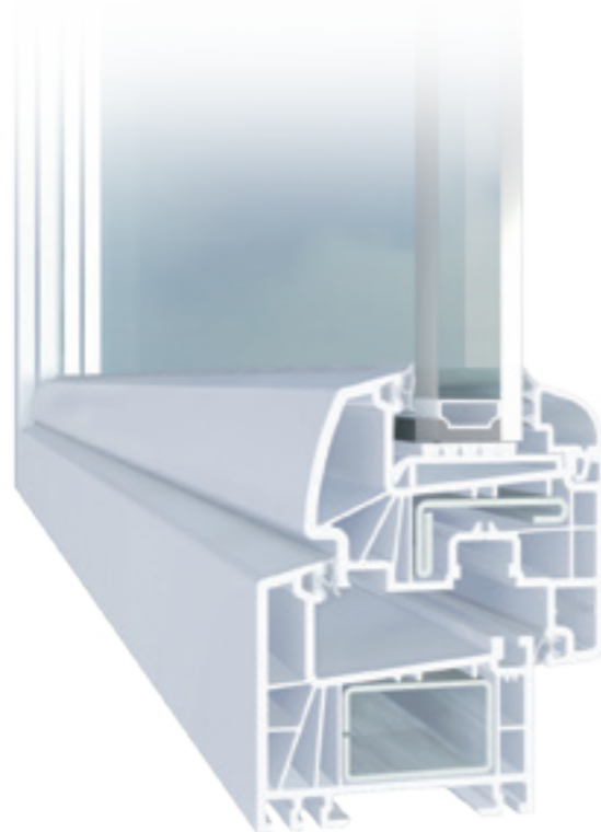
Coupe d'angle de fenêtre
